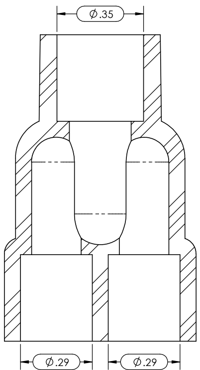
SECTION A-A SCALE 4 : 1
