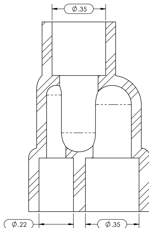
SECTION A-A SCALE 4 : 1
