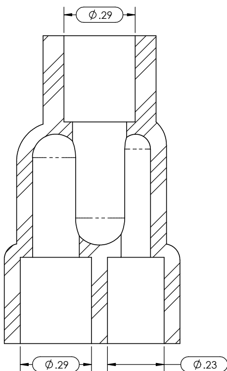
SECTION A-A SCALE 4 : 1
