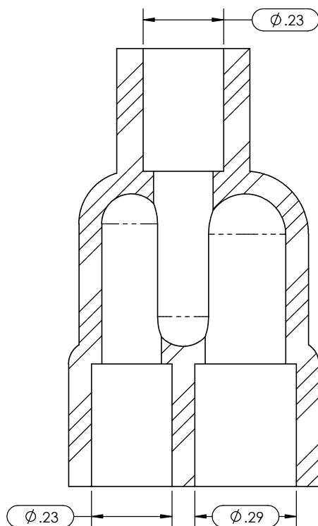
SECTION A-A SCALE 4 : 1
