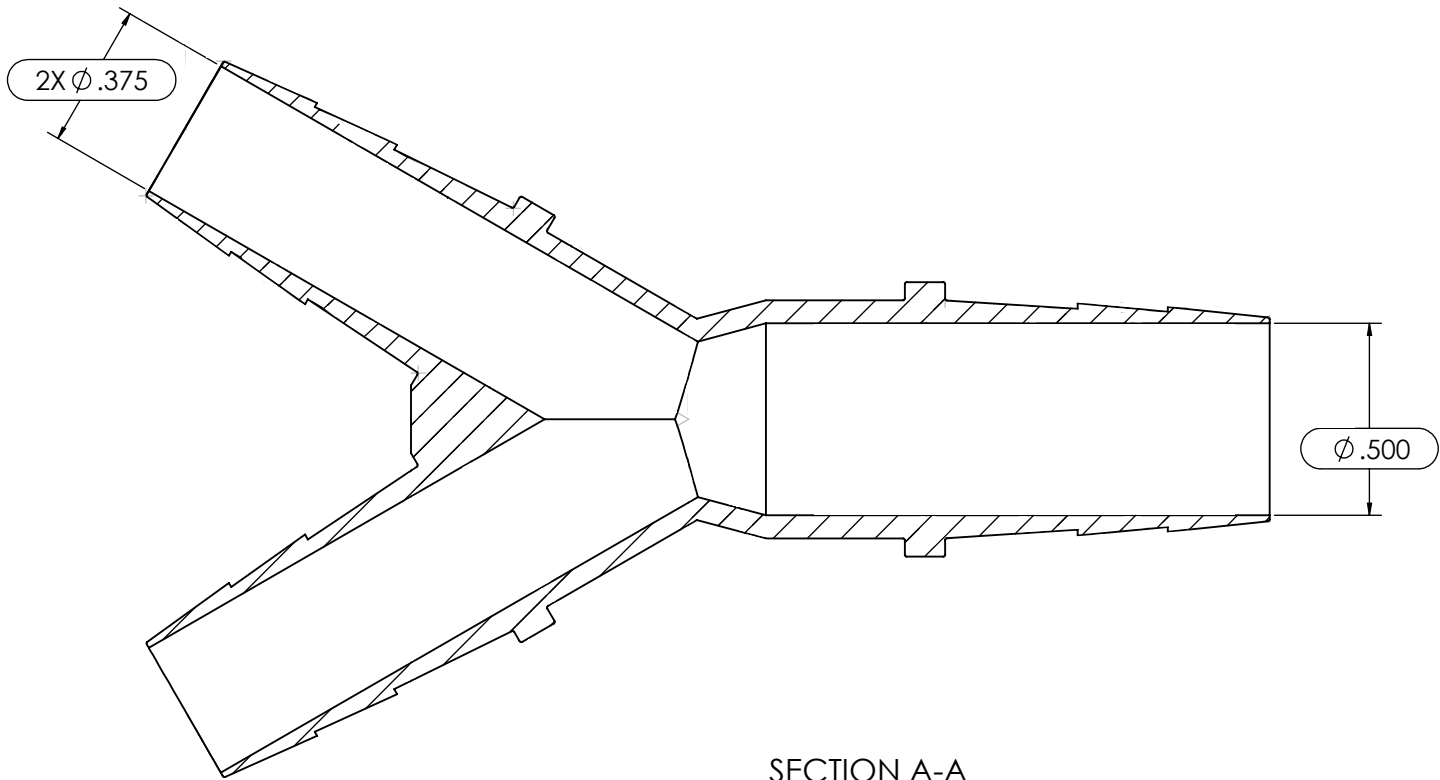
SECTION A-A
